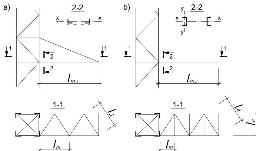
Hình 21 – Sơ đồ xà ngang
