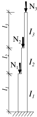
Hình D.2 – Sơ đồ cột
