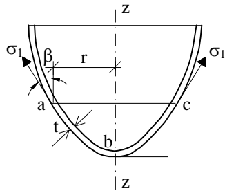
Hình 15 – Sơ đồ vỏ tròn xoay
