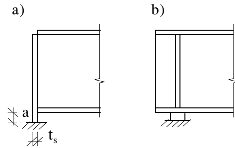
Hình 12 – Sơ đồ đặt sườn cứng ở gối
