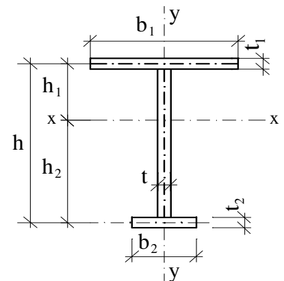
Hình E.1 – Sơ đồ dầm tiết diện chữ I có một trục đối xứng có l_0/b_2 > 25 .
