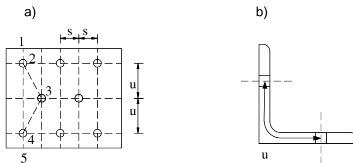
Hình 1 – Cách xác định diện tích thực
