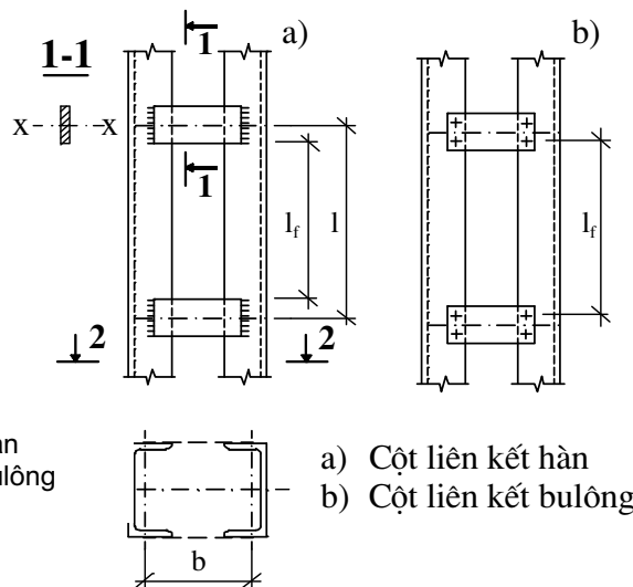
Hình 5 – Cột tổ hợp bằng bản giằng
